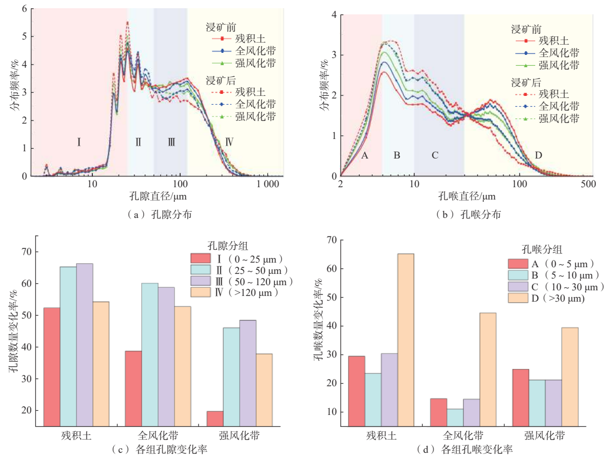
图 5 不同风化带稀土矿试样孔隙、孔喉变化曲线
