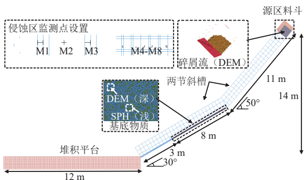
图 4 大型物理试验数值模型
