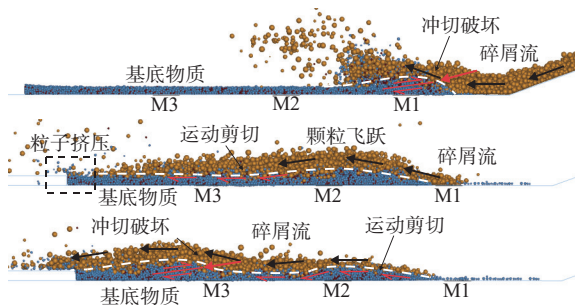
图7 碎屑流动力侵蚀过程
