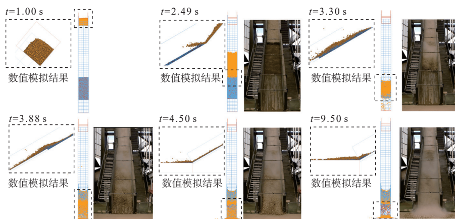
图6 数值模拟和试验结果对比图
