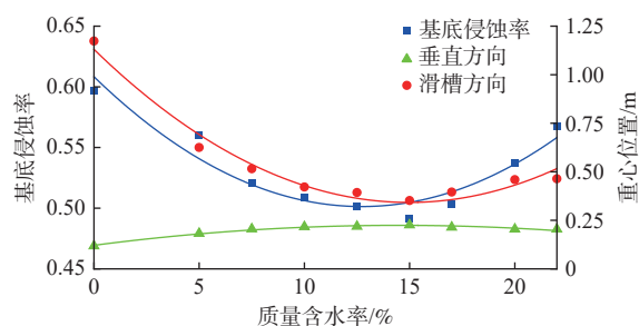
图10 侵蚀、堆积与含水率关系曲线
