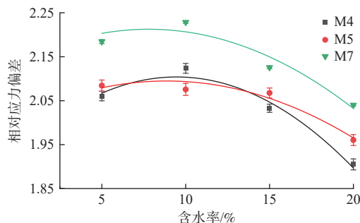
图 12 相对应力偏差与含水率关系曲线
