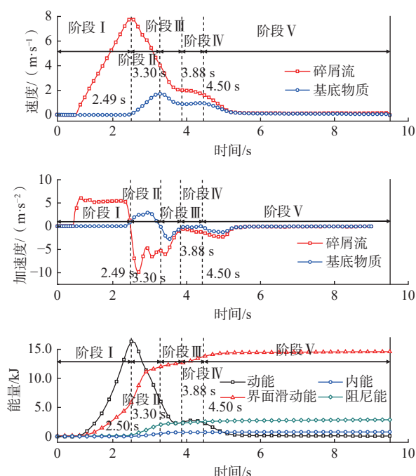
图5 速度、加速度、能量的时间演化曲线
