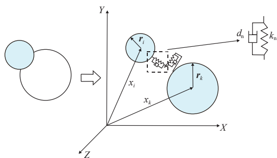
图2 离散单元法接触模型
