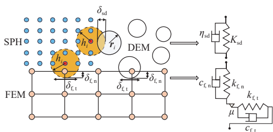
图3 SPH-DEM-FEM耦合接触模型
