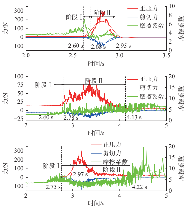
图8 监测点受力时间演化曲线
