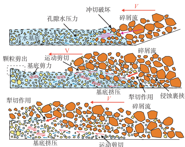
图9 碎屑流动力侵蚀效应宏观作用机制
